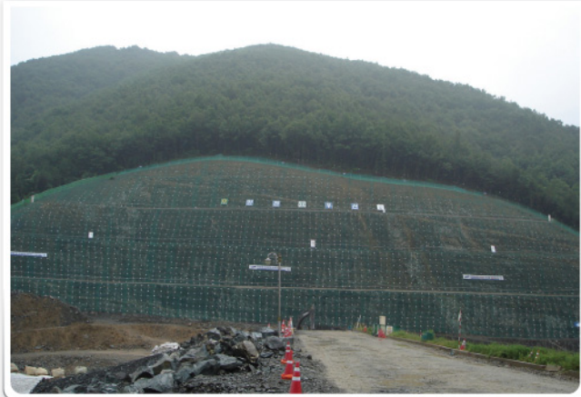
강관 보강형 다단 그라우팅
